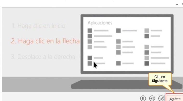
Figura 9. Instalación Office 365
